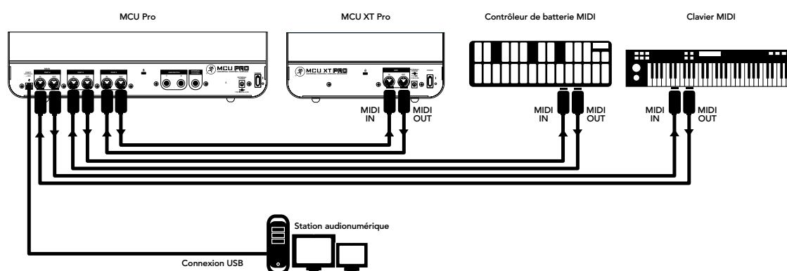
Plan 3 : Avec plusieurs périphériques MIDI
